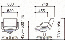
ME-4085LV
