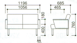
LA70-2BF・LA70-2BV
