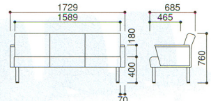
LA70-3BF・LA70-3BV
