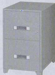
29-0055-0 EB4-2 (オールロック式) ¥226,800 (¥216,000) 29-0056-0 EB4-2C (各段シリンダー式) ¥241,185 (¥229,700) 外寸法/W517×D760×H827mm 引出内寸法/W388×D646×H300mm ■仕切板4枚付 質量/155kg
