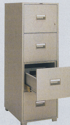
53-0027-0 B4-4A (オールロック式) ¥491,400 (¥468,000) 外寸法/W547×D795×H1618mm 引出内寸法/W390×D633×H303mm ■仕切板8枚付 質量/387kg 引出内容量/75ℓ
