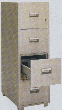
53-0025-0 A4-4A (オールロック式) ¥437,850 (¥417,000) 外寸法/W482×D795×H1462mm 引出内寸法/W325×D633×H264mm ■仕切板8枚付 質量/340kg 引出内容量/54ℓ
