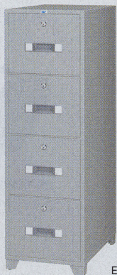
29-0053-0 EA4-4 (オールロック式) ¥397,215 (¥378,300) 29-0054-0 EA4-4C (各段シリンダー式) ¥425,985 (¥405,700) 外寸法/W460×D760×H1451mm 引出内寸法/W331×D646×H275mm ■仕切板8枚付 質量/260kg
