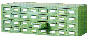
26-0789-0 TU-484 ¥139,125 (¥132,500) トレー内寸/W123×D388×H65mm ■仕切板32枚付 ■質量/62kg
