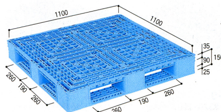
55-0030-0 (パレット)D4-1111-3 ¥9,555 (¥9,100)
