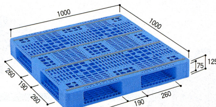
55-0019-0 (パレット)R4-1010-2 ¥16,275 (¥15,500)
