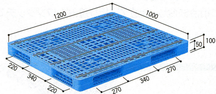
55-0017-0 (パレット)R4-1012-4 ¥14,805 (¥14,100)
