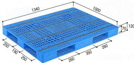
55-0018-0 (パレット)R4-100134 ¥15,960 (¥15,200)
