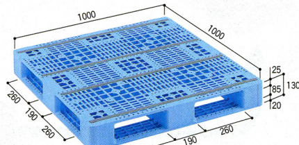
55-0020-0 (パレット)D4-1010-3 ¥15,120 (¥14,400)
