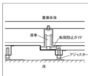
下部レール構造
