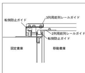
上部レール構造
