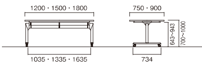
■アジャスト機能付キャスター キャスター上部のリングにより高さ調節できます。制動力の高いリフトロック式ストッパーです。
