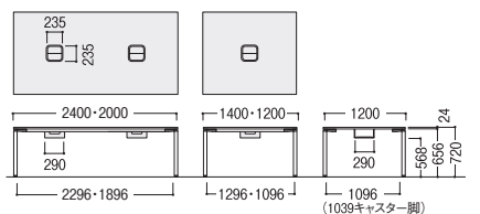
NTS-2412-2012NT(C) NTS-1412-1212NT(C)
