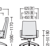
TLKE-6N/L
