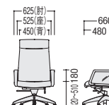
TLKE-H8N/L
