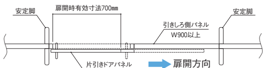
片引きドア取付例 (右引き扉)
