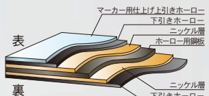
板面 断面図
