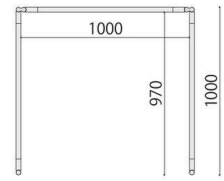
QSB説明(レイアウト寸法図)
