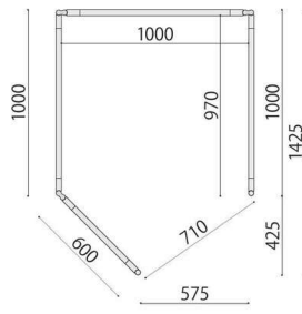
QSB説明(レイアウト寸法図)
